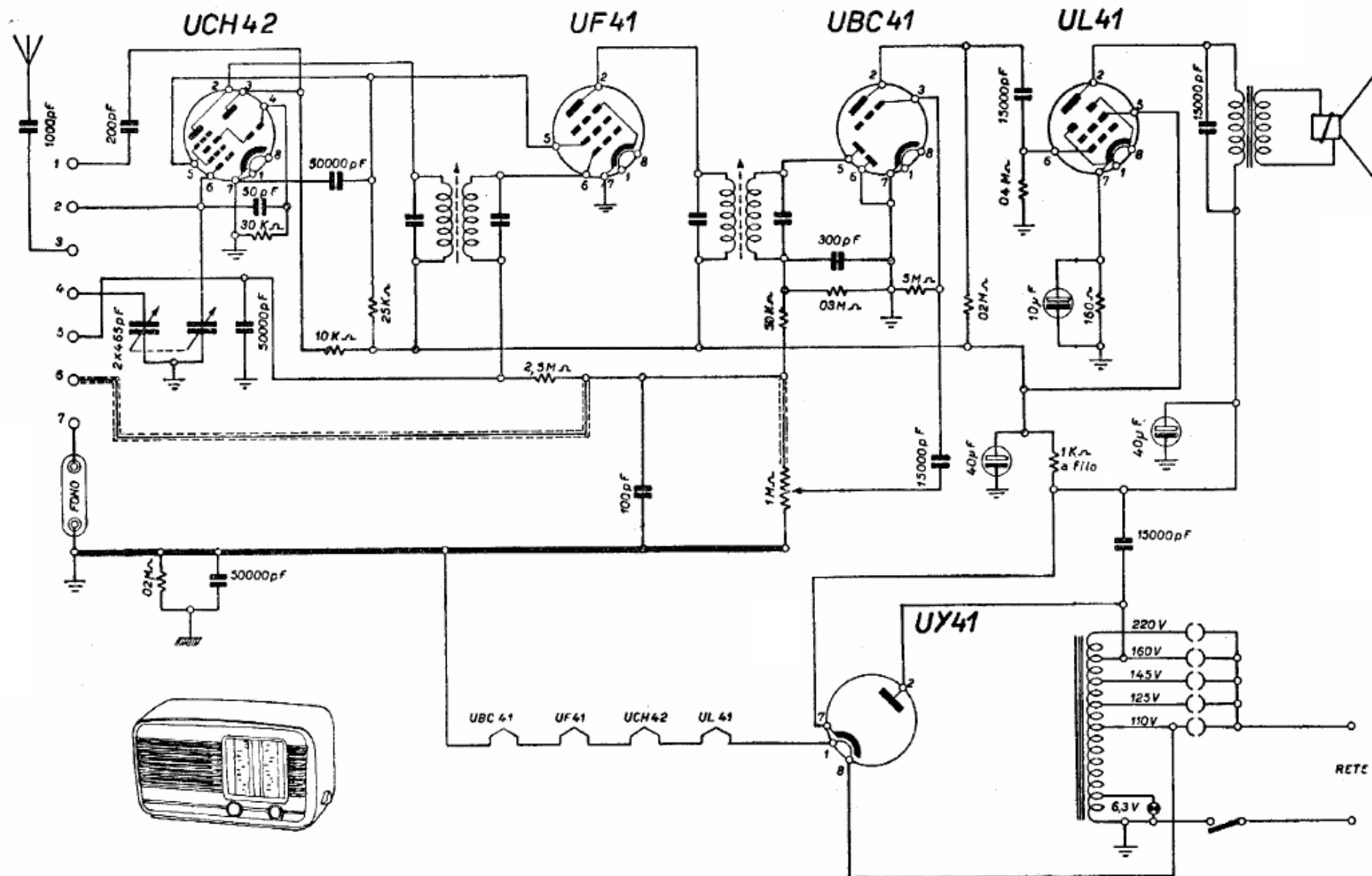
REOM - Sintomagic Radio mod. n0 - Ricevitore ad onde medie e corte. Media frequenza 470 ke. Valvole serie rimlock. Potenza d'uscita 2 watt. Consumo 40 watt.
